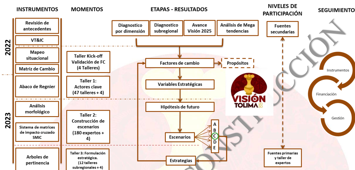
Ilustración 19 Esquema metodológico
